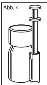
Abb. 4: Um die Pipette an der Flasche zu befestigen, nehmen Sie die beliebige Halterung und ziehen Sie die Klebefolie ab. Kleben Sie nun die Halterung senkrecht an die Flasche, so dass die Standfüßchen der Halterung nach unten zeigen und die Öffnung nach oben gerichtet ist. Stellen Sie die ausgespülte und abgetrocknete Pipette in die Halterung, Pipette und Halterung bilden nun eine Einheit.
